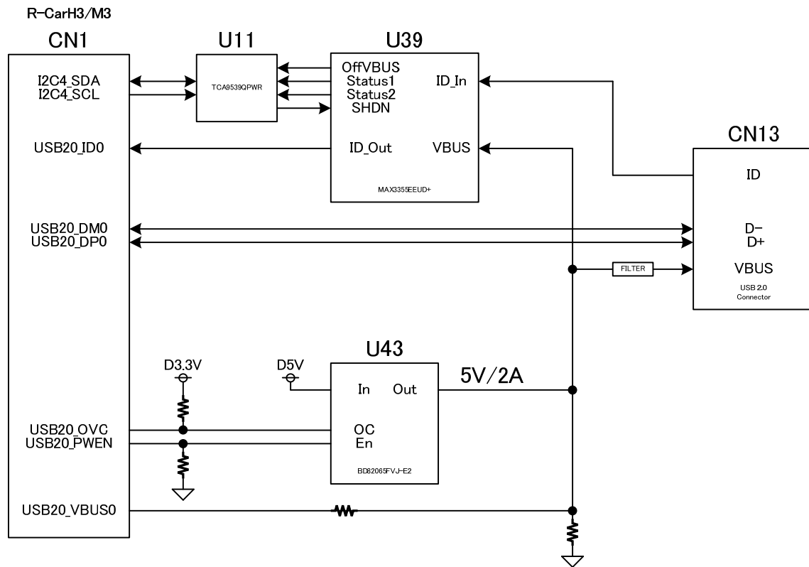
Figure 4-5 : USB 2.0 I/F
